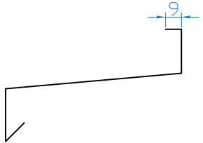
Gesimsblech (GB)
