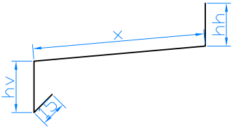
Fensterblech (FB)
